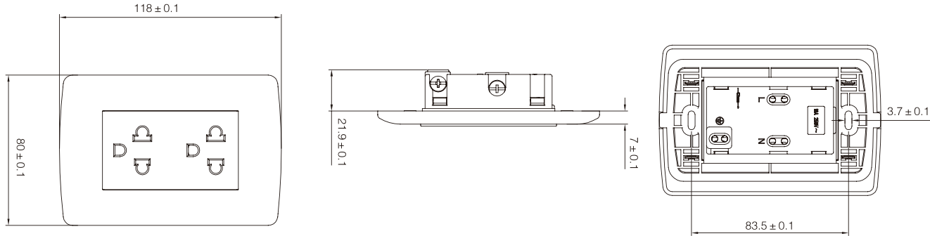
LP1006 6G Plate
